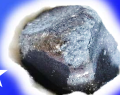
アエンデ隕石
